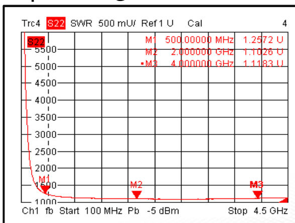
Output VSWR @+85°C
