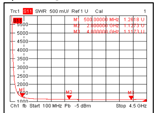
Input VSWR @+85°C
