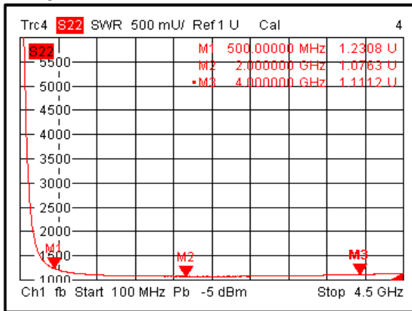
Output VSWR @-40°C
